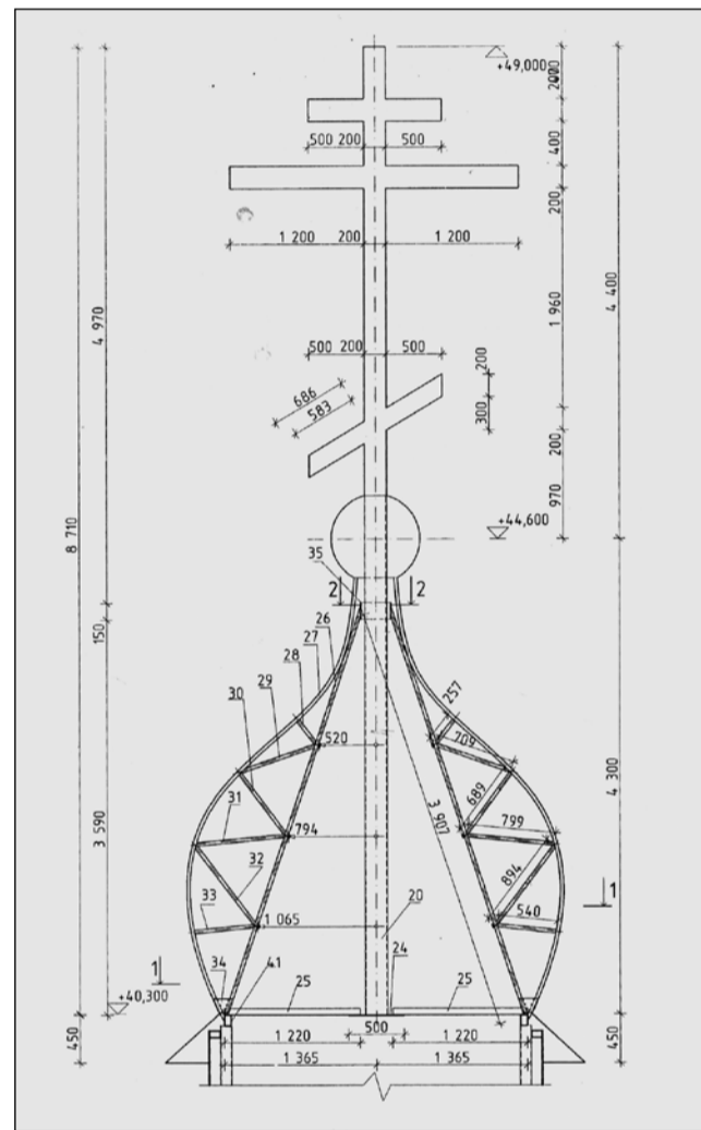
Рабочий чертёж Креста и центральной главки
